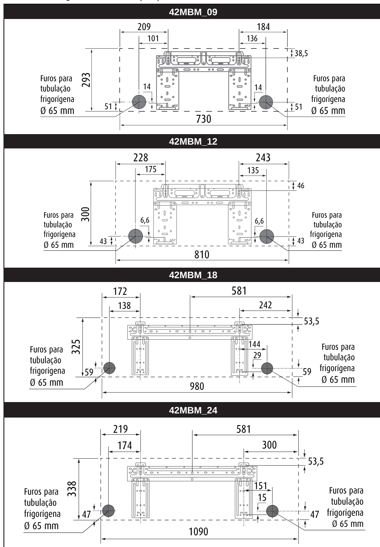
FIG. 14- PLACAS DE MONTAGEM
