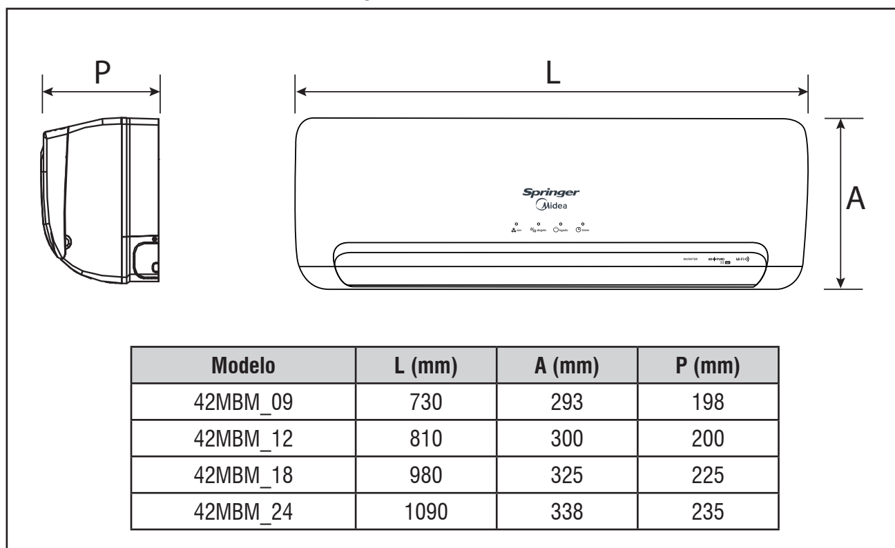
FIG. 13 - DIMENSIONAL DAS UNIDADES EVAPORADORAS
