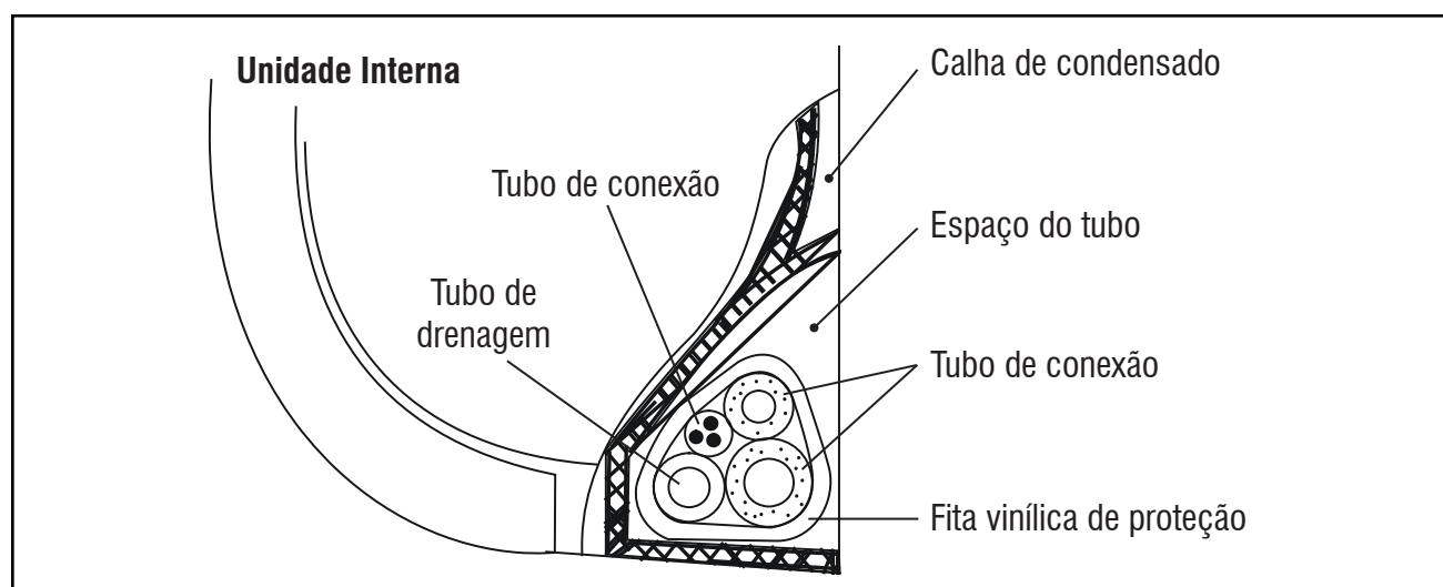
FIG. 10 - TUBOS DE CONEXÃO E DRENAGEM
