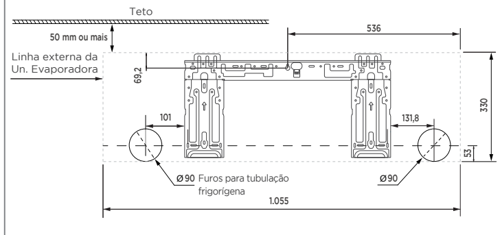
FIG. 18b - SUPORTES DE MONTAGEM
