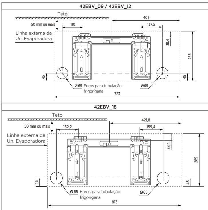
FIG. 18a - SUPORTES DE MONTAGEM
