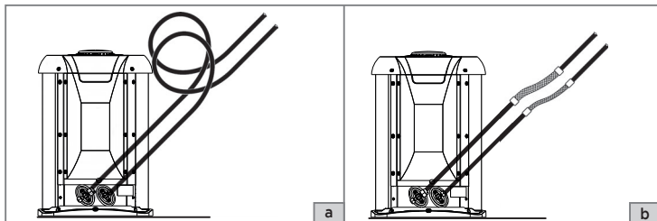
FIG. 20 - LOOP'S E TUBOS FLEXÍVEIS
