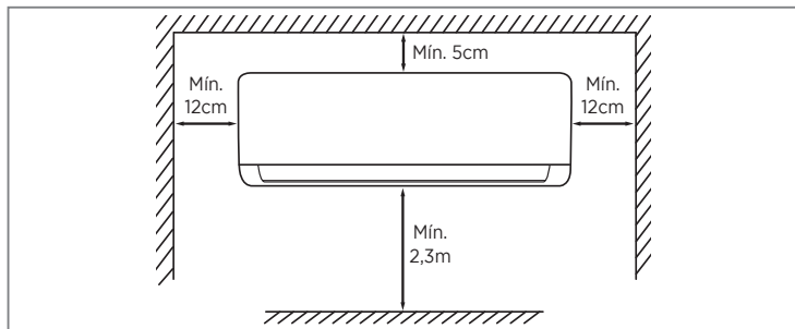
FIG. 6 - ESPAÇAMENTOS MÍNIMOS RECOMENDADOS
