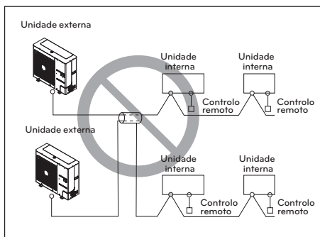
Cabo multi-núcleo
