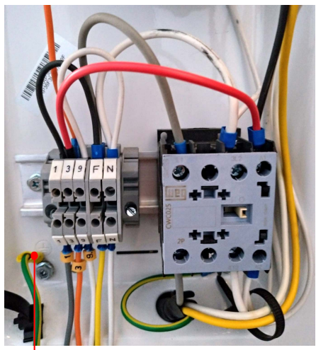
Aterramento Unidade Externa
