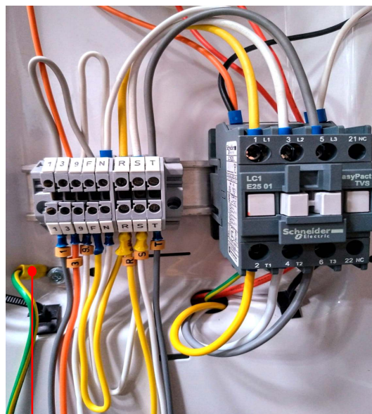
Aterramento Unidade Externa
