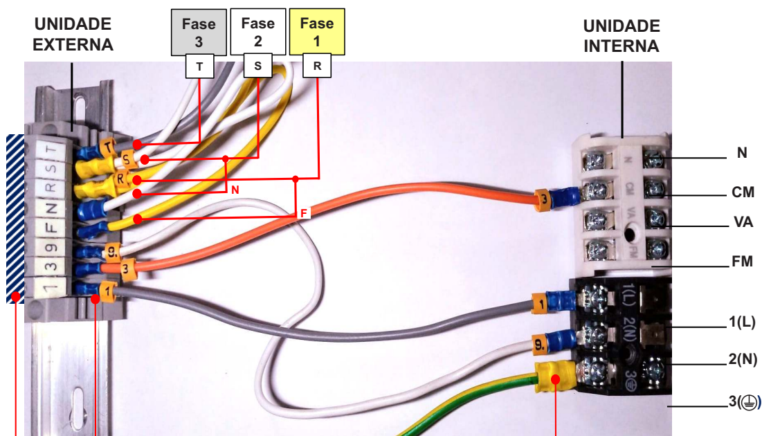
Ligação Realizada em Campo
