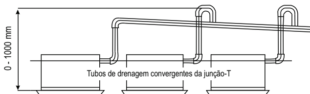
Tubos de drenagem convergentes da junção-T
