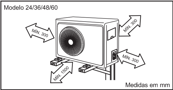
DISTÂNCIAS PARA FIXAÇÃO DA BASE DA UNIDADE CONDENSADORA
