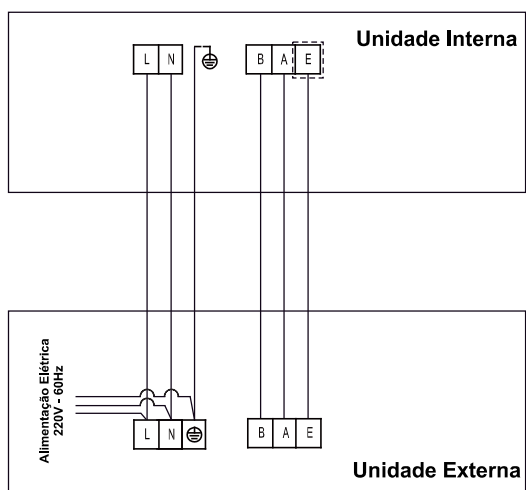
Esquema de ligação das unidades CASSETE (KX) Modelo 48/60 - 220V ~60Hz - (FRIO)
