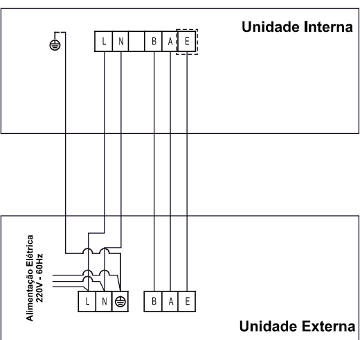
Esquema de ligação das unidades PISO-TETO (PX) Modelo 48/60 - 220V ~60Hz - (FRIO)
