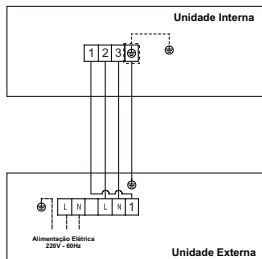
Esquema de ligação das unidades PISO-TETO (PX) Modelo 24 - 220V ~60Hz - (FRIO)
