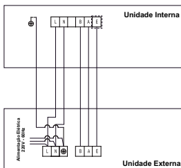
Esquema de ligação das unidades PISO-TETO (PX) Modelo 48/60 - 220V ~60Hz - (FRIO)
