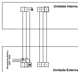
Esquema de ligação das unidades CASSETE (KX) Modelo 48/60 - 220V ~60Hz - (FRIO)
