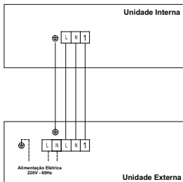
Esquema de ligação das unidades CASSETE (KX) Modelo 24 - 220V ~60Hz - (FRIO)
