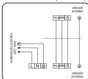
Esquema de ligação de unidades Piso-Teto modelos 48/60 - 220V ~ (Somente frio)
