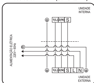
Esquema de ligação de unidades Piso-Teto modelos 36 - 220V ~ (Somente frio)
