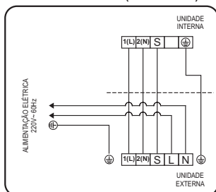
Esquema de ligação de unidades Cassete modelo 36 - 220V ~ (Somente frio)
