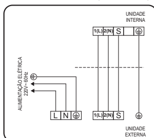
Esquema de ligação de unidades Cassete modelos 48/60 - 220V ~ (Somente frio)
