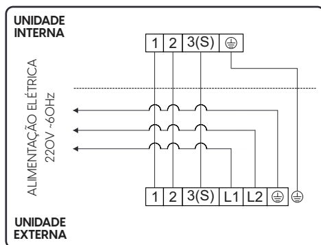
Esquema de interligação de unidades modelo 36.000 - 220V - 60Hz (Frio e Quente/Frio)
