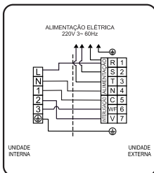
Esquema de ligação das unidades modelo 48,000 • 220V 3~ 60Hz (Quente/Frio)
