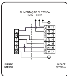
Esquema de ligação das unidades modelo 48,000 • 220V 3~ 60Hz (Quente/Frio)
