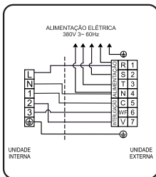
Esquema de ligação das unidades modelo 48,000 • 380V 3~ 60Hz (Quente/Frio)
