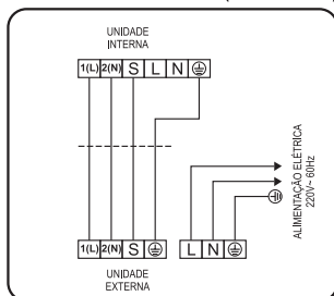
Esquema de ligação de unidades Cassete modelo 36/60.000 - 220V ~ (Somente frio)
