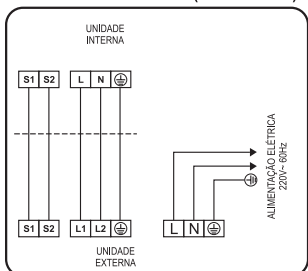
Esquema de ligação de unidades Cassete modelo 48.000 - 220V ~ (Somente frio)
