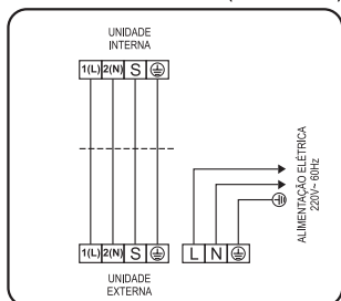
Esquema de ligação de unidades Piso-Teto modelo 36/60.000 - 220V ~ (Somente frio)
