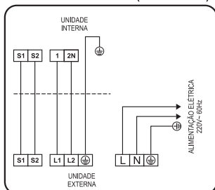
Esquema de ligação de unidades Piso-Teto modelo 48.000 - 220V ~ (Somente frio)
