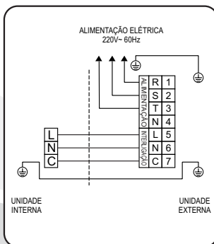
Esquema de ligação de unidades modelo 48.000 - 220V 3~ (Somente frio)
