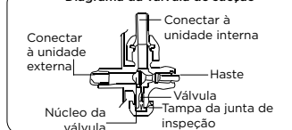
Diagrama da válvula de sucção
