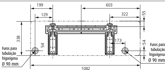
FIG. 11 - PLACAS DE MONTAGEM
