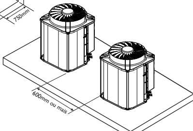
FIG. 4 - ESPAÇAMENTOS MÍNIMOS RECOMENDADOS
