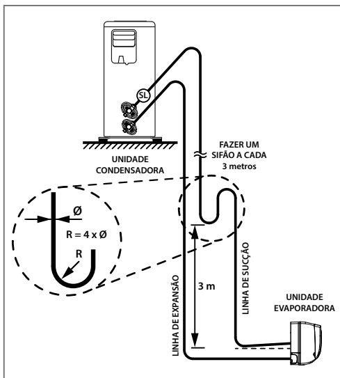
FIG. 12 - LINHAS DE INTERLIGAÇÃO
