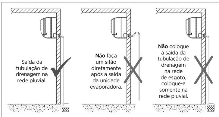
FIG. 7 - EXEMPLOS DE SITUAÇÕES DE DRENAGEM
