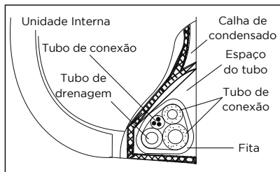
FIG. 8 - TUBO DE CONEXÕES
