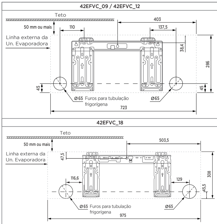
FIG. 18a - SUPORTES DE MONTAGEM
