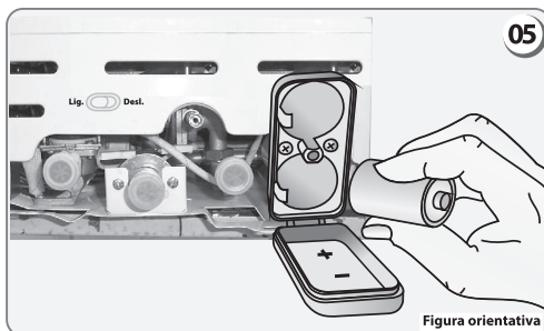
Figura orientativa
