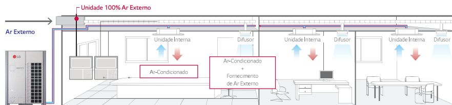
Unidade Externa MULTI V 5
