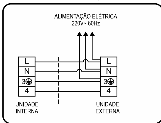
Esquema de ligação de unidades Modelos 09/12/18/24/30/36.000 (FRIO e QUENTE/FRIO)
