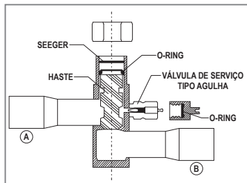
FIG. 21 - VÁLVULA DE SERVIÇO FECHADA
