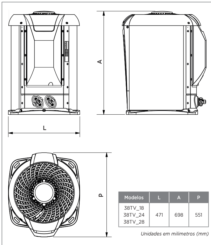
FIG. 9 - DIMENSIONAIS
