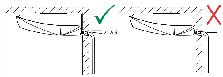
FIG. 15 - INCLINAÇÃO DRENAGEM
