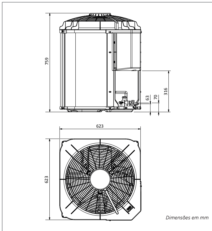
FIG. 7 - DIMENSIONAL UNIDADES CONDENSADORAS
