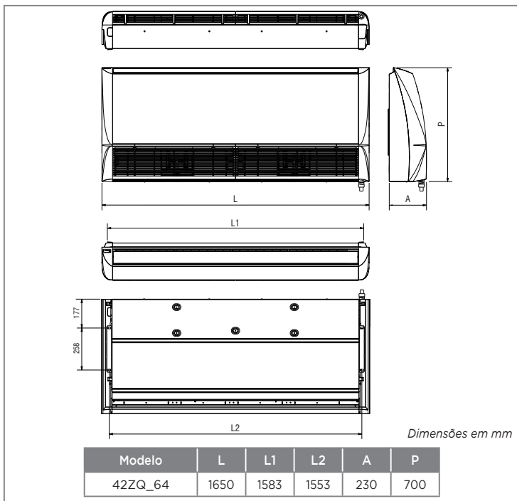
FIG. 8 - DIMENSIONAL UNIDADES EVAPORADORAS
