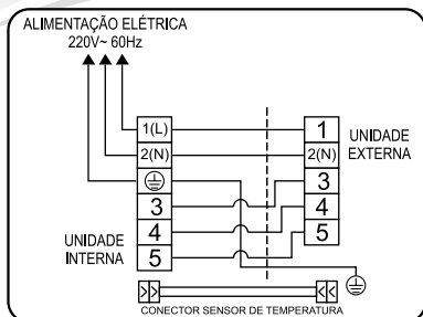
Esquema de ligação de unidades modelo 24.000 - Quente/Frio - 220V~
