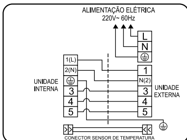
Esquema de ligação de unidades modelo 30.000 - Quente/Frio - 220V~
