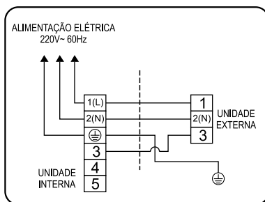
Esquema de ligação de unidades modelo 24.000 - Frio - 220V~
