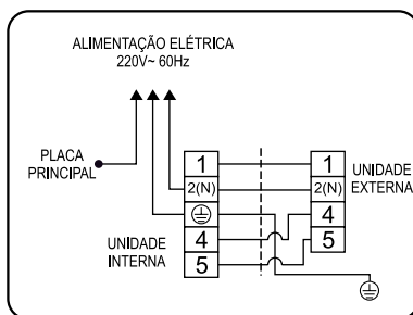
Esquema de ligação de unidades modelo 9/12/18.000 - Quente/Frio - 220V~
