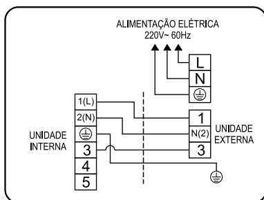
Esquema de ligação de unidades modelo 30.000 - Frio - 220V~
