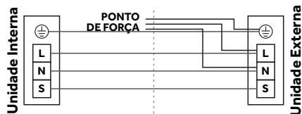
ICS 24K Quente e Frio
