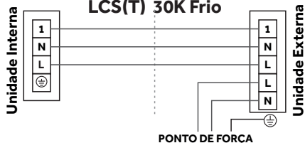
LCS(T) 30K Frio
