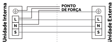
ICST 12K Quente e Frio
