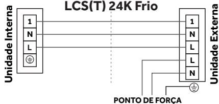
LCS(T) 24K Frio
