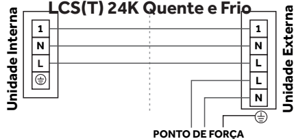
LCS(T) 24K Quente e Frio
